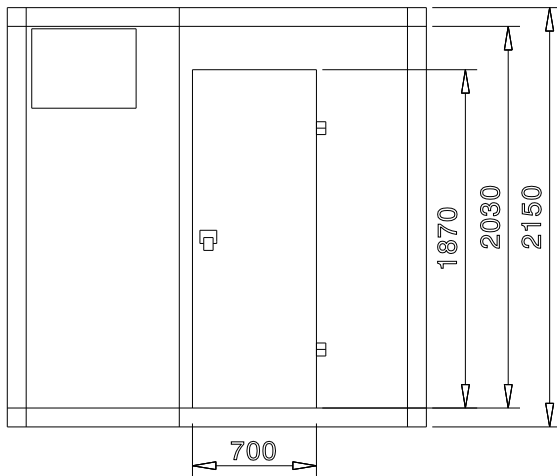
Zij aanzicht
